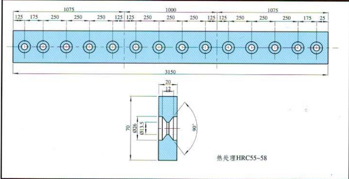
Q6.35 × 3100 剪板机刀片
