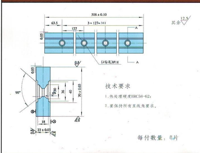
Q11-6.3 × 2000 剪板机刀片
