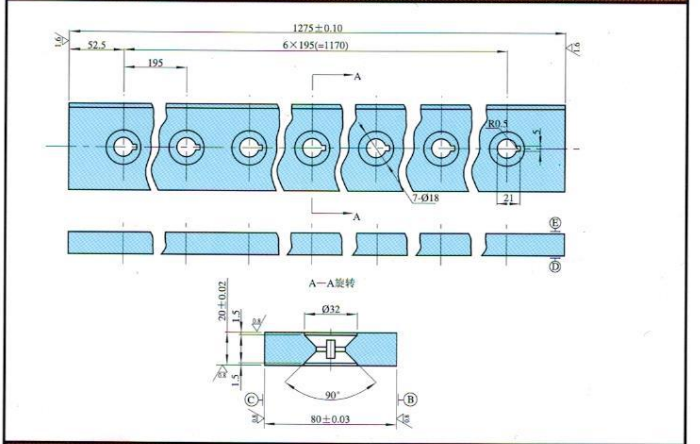
QC12Y-8 × 5000 液压摆式剪板机下刀片
