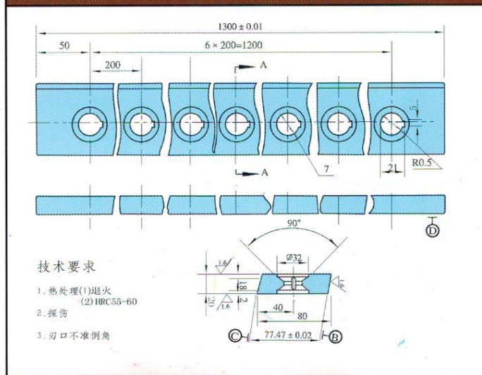
QC12Y-4 × 2500 剪板机刀片
