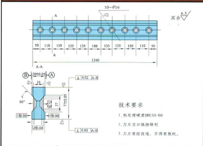
Q11-3.5 × 1300 剪板机刀片
