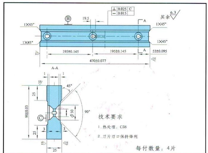
Q11-3 × 1800 剪板机刀片
