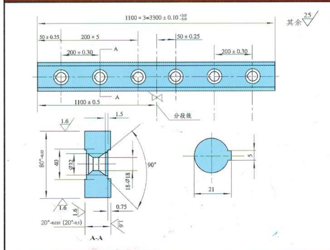
6 × 3200 剪板机下刀
