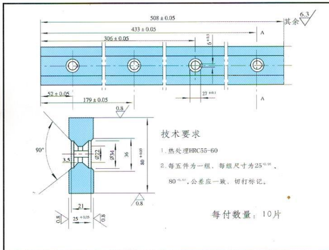
Q11-6 × 2500 剪板机刀片
