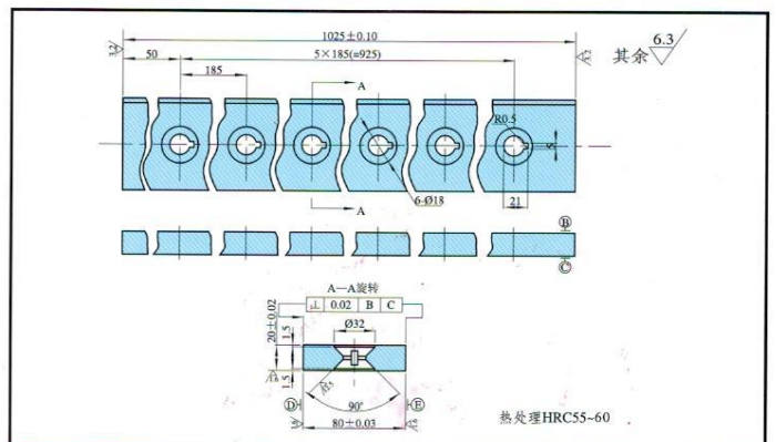
Q12Y-6 × 4000 液压摆式剪板机刀片
