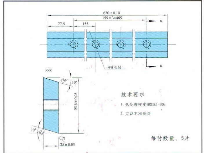
DLB-12 × 3050 剪板机上刀片
