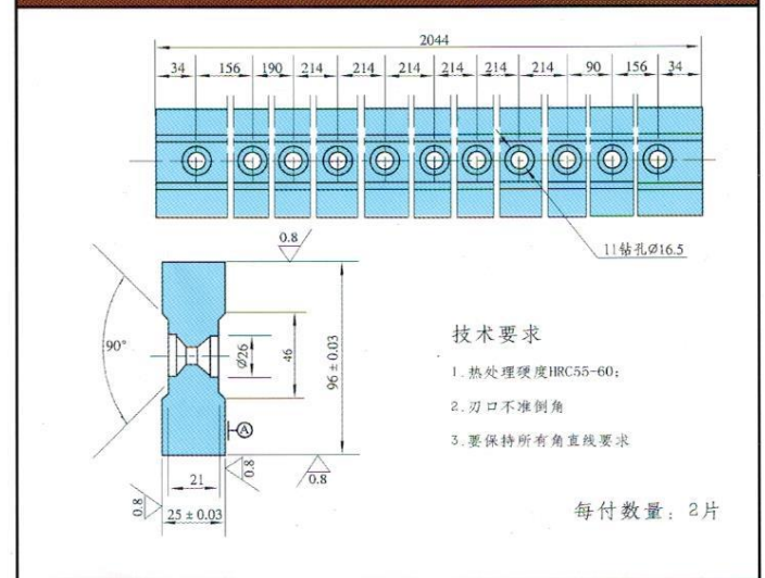
Q11-7 × 2000 剪板机刀片
