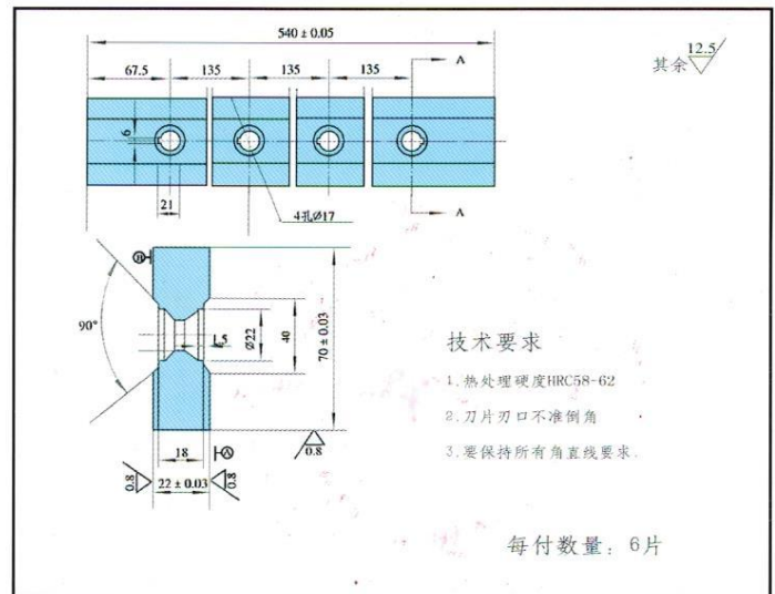
Q11-2.5 × 1600 剪板机刀片
