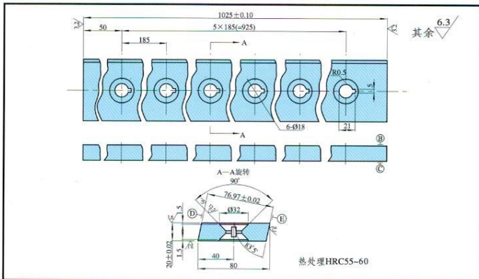
QC12Y-6 × 4000 液压摆式剪板机刀片
