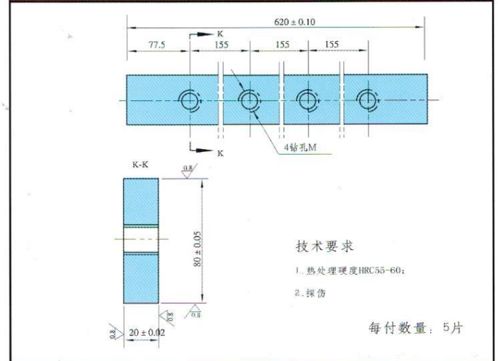
DLB-12 × 3050 剪板机下刀片
