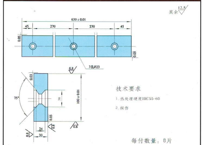
Q12-20 × 2500 剪板机刀片
