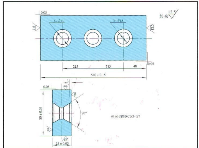
12 × 2000 剪板机刀片
