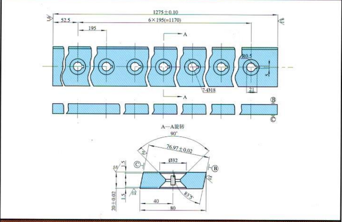
QC12Y-8 × 5000 液压摆式剪板机上刀片
