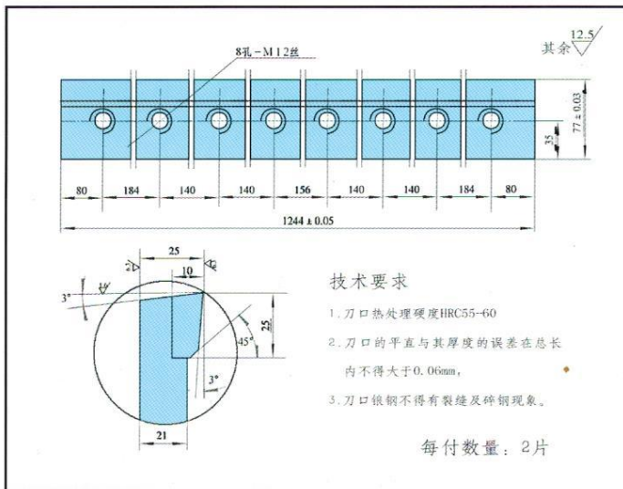
Q11-3 × 1200 剪板机刀片
