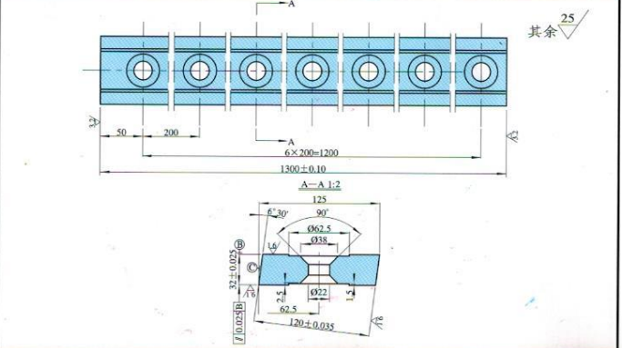
QC12Y-20 × 2500C 剪板机上刀片
