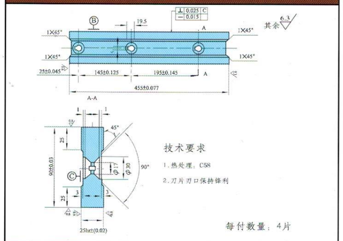
Q11-3 × 1800 剪板机刀片
