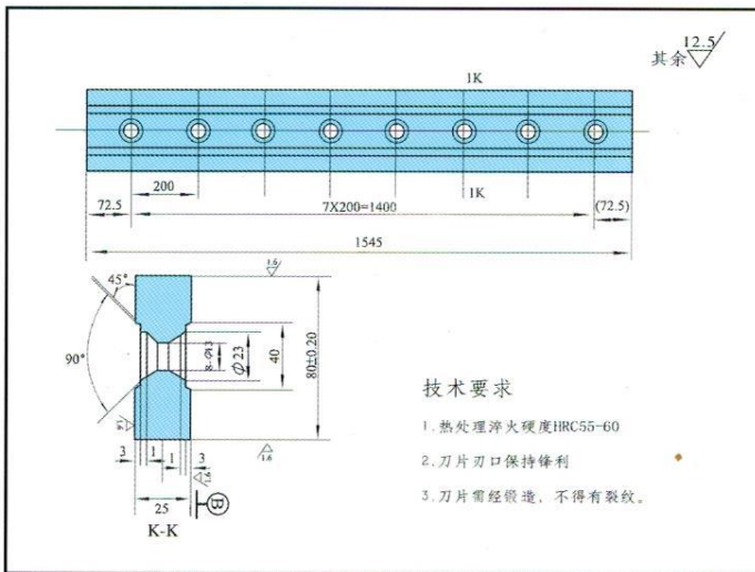
Q11-3 × 1500 剪板机刀片
