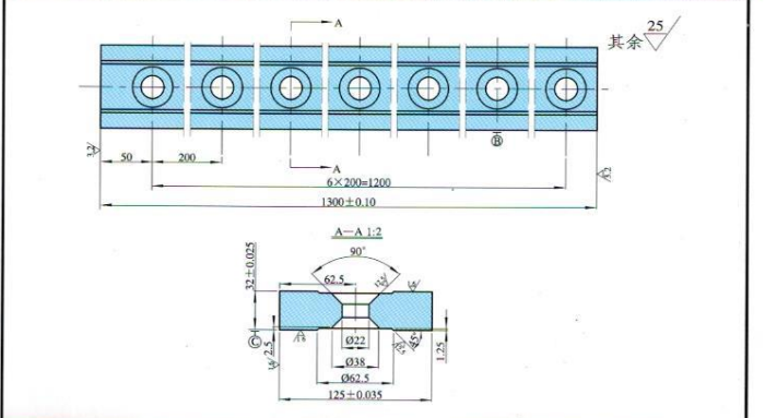
QC12Y-20 × 2500C 剪板机下刀片
