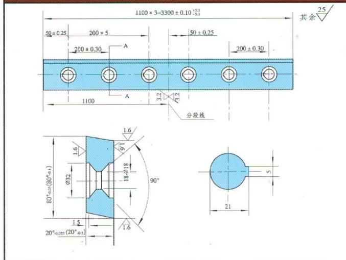
6 × 3200 剪板机上刀
