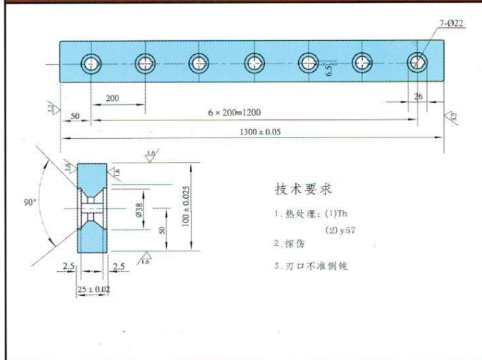
QC12Y-12 × 2500 剪板机下刀片
