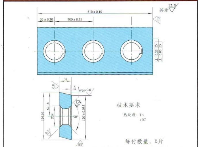
20 × 4000 剪板机上刀
