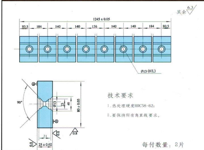
Q11-3 × 1200 剪板机刀片
