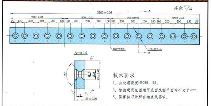
LVD-(HD)-13 × 3100 剪板机刀片
