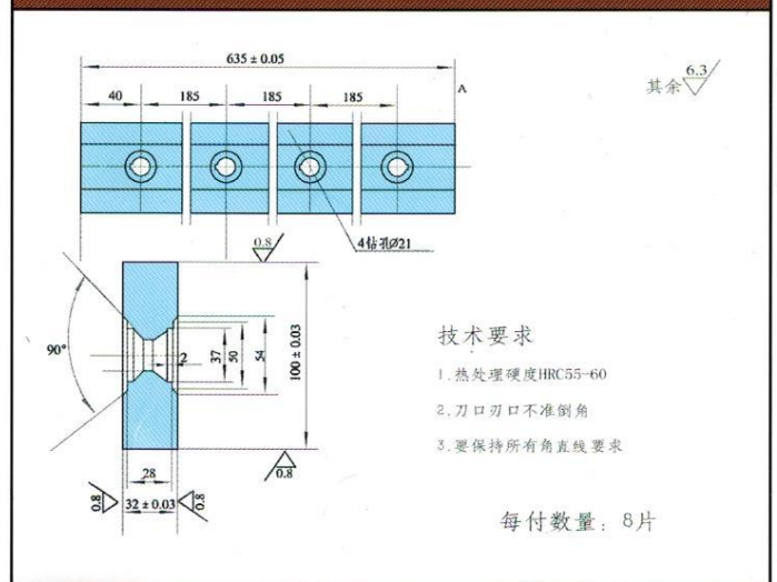
Q11Y-20 × 2500 剪板机刀片
