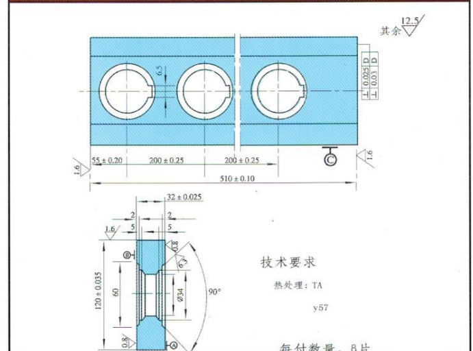
20 × 4000 剪板机下刀
