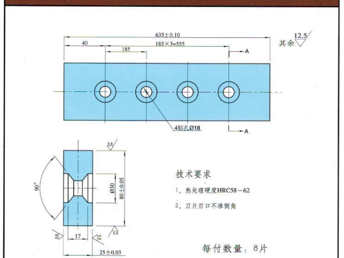
Q11-3 × 1800 剪板机刀片
